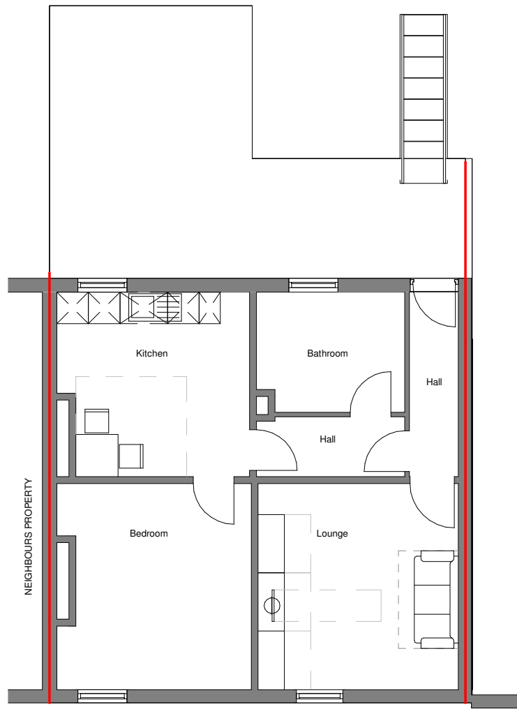
02 | Level 1 1 : 100
