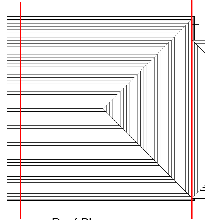
03 | Roof Plan 1 : 100
