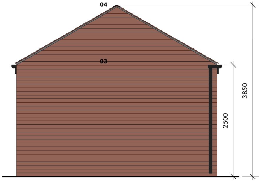
elevation a
