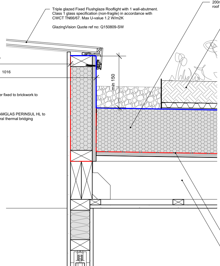
02 Pullout detail 1:5 @ A3
