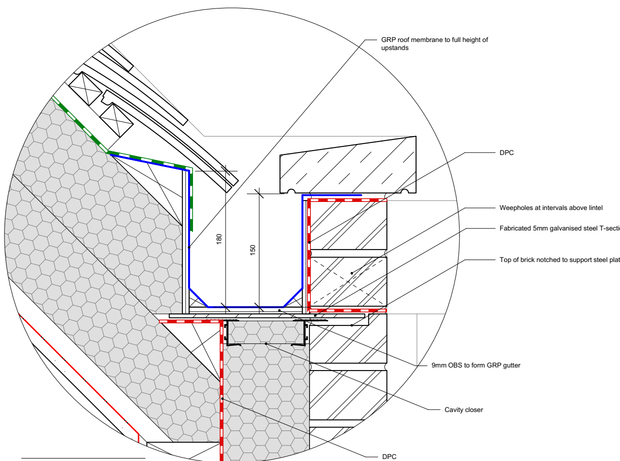
02 Pullout detail 1:5 @ A3
