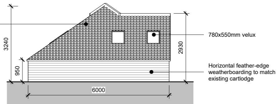
Elevation B 1 : 100
