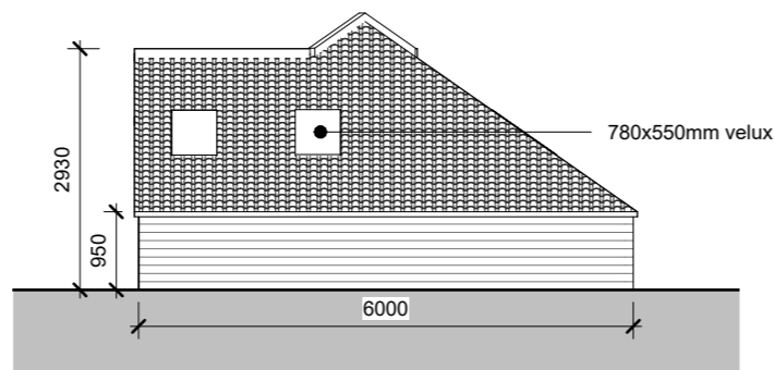
Elevation C 1 : 100
