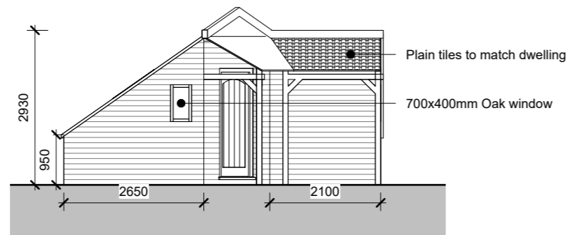
Elevation A 1 : 100
