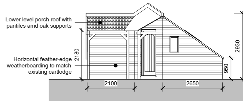
Elevation D 1 : 100
