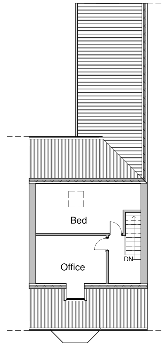
4 Loft 1 : 100
