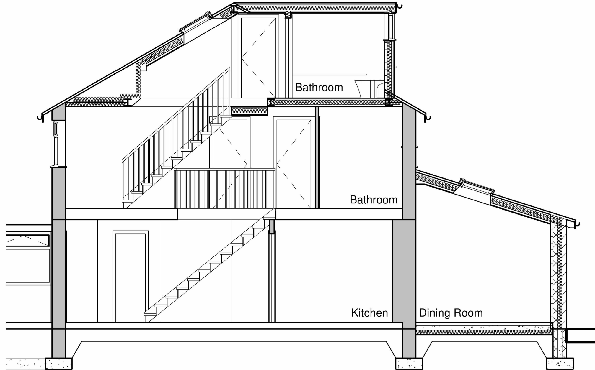
1 Section 2 1 : 50
